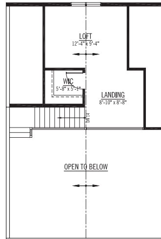
LOFT
